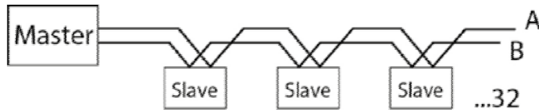
Diagram 4: RS485 haberleşme şeması
