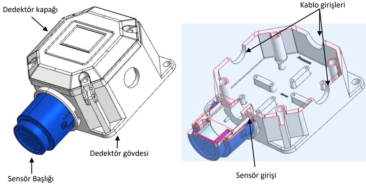
Diagram 1: Dedektör gövdesi
